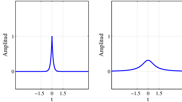
FIGURA 5. La función g(x) = e^{-2\pi|x|} y su transformada
