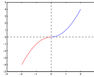
FIGURA 2. Simetría impar para f(x) = x^2 en x \in (0, 2)
