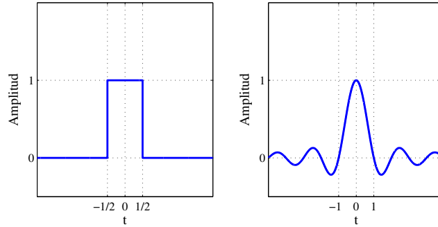
FIGURA 4. Pulso rectangular y su transformada
