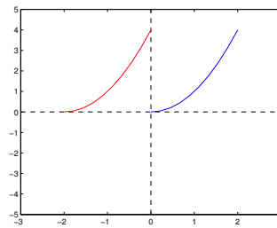
FIGURA 3. Traslación para f(x) = x^2 en x \in (0, 2)
