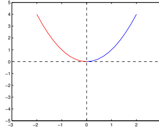
FIGURA 1. Simetría par para f(x) = x^2 en x \in (0, 2)
