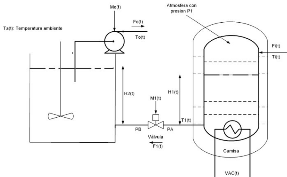
Figura 2.1: Diagrama del proceso
